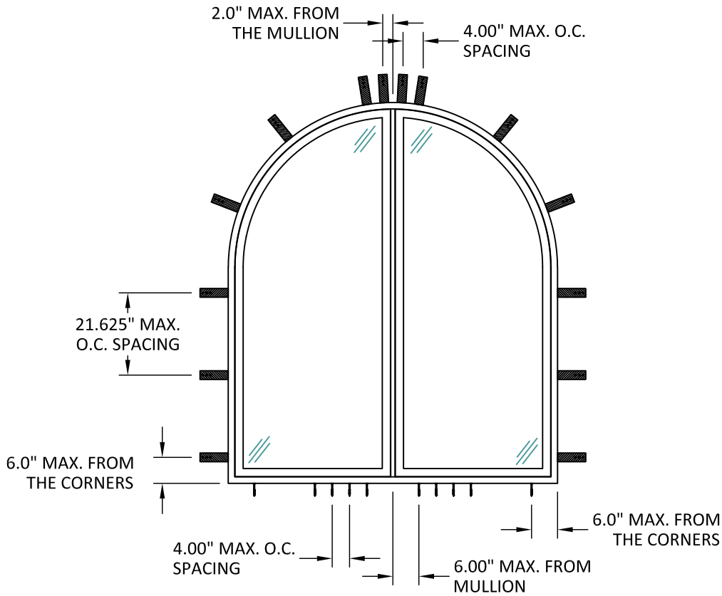
ELEVATION
