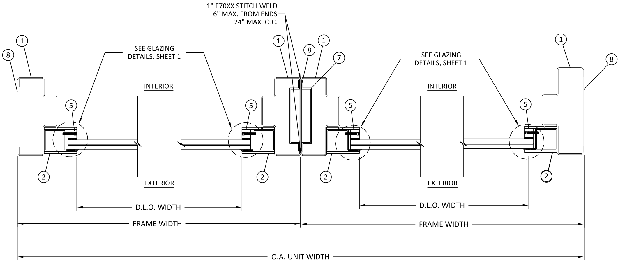
A HORIZONTAL SECTION 7 JAMB
