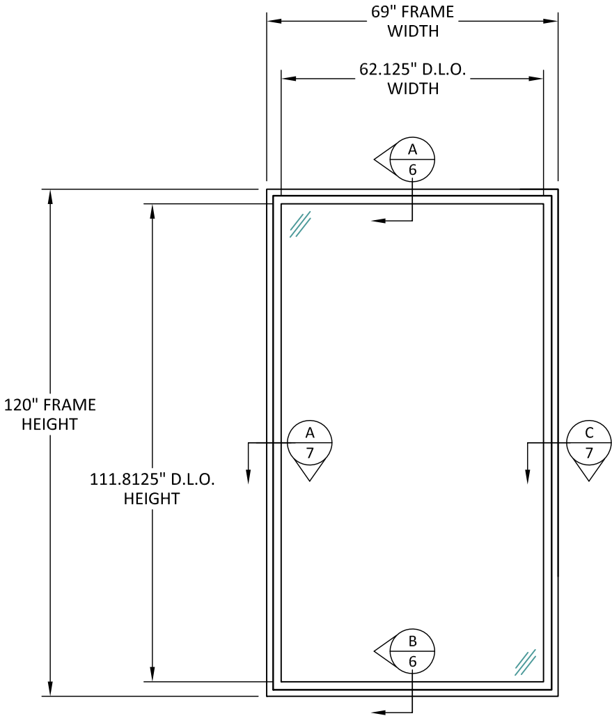
ELEVATION
